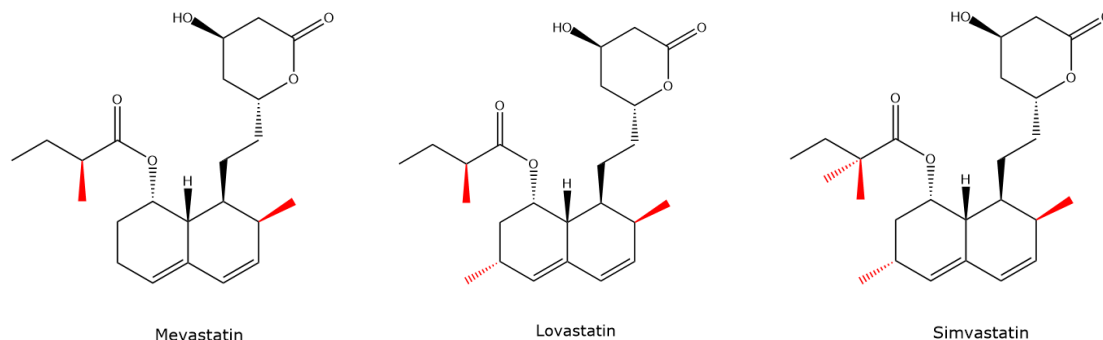
Slika 5. Strukturni prikaz Mevastatina, Lovastatina i Simvastatina s crveno označenim metilnim skupinama.
