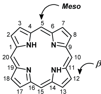
Slika 4. Struktura porfirina (16).
