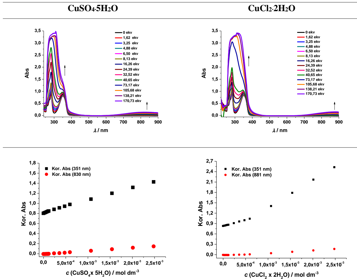
Slika 147. UV/Vis spektri titracije spoja 4a ( c_0 = 1,50 \cdot 10^{-5} \text{ mol/dm}^3 ) s \text{CuSO}_4 \cdot 5\text{H}_2\text{O} i \text{CuCl}_2 \cdot 2\text{H}_2\text{O} te pripadajući maksimumi apsorbancije (351 nm i maksimum kompleksa)
