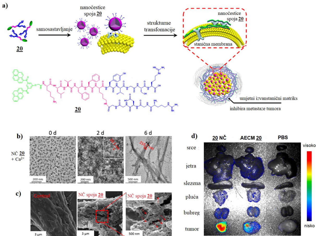
Slika 29. (a) struktura i shematski prikaz transformacije nanočestica konjugata 20 u nanovlakna, (b) TEM slike morfolofije transformacije nanočestica konjugata 20 u prisutnosti iona \text{Ca}^{2+} u vodenoj otopini, (c) SEM slike strukturalne transformacije nanočestica konjugata 20 na površini stanice, (d) ex vivo fluorescencijske slike biodistribucije konjugata 20 u različitim tkivima i tumoru 103
