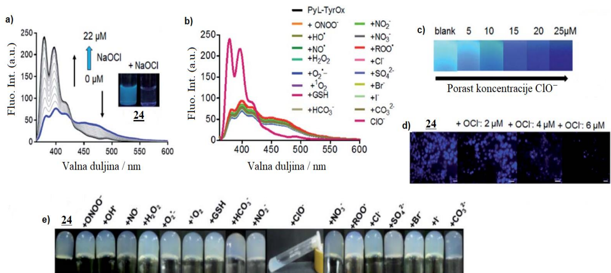
Slika 32. (a) emisijski spektar titracije spoja 24 (20 μM, \lambda_{\text{ex}} = 345 \text{ nm} ) s ionima \text{ClO}^- (0 – 22 μM), (b) promjene u emisijskom spektru spoja 24 (20 μM, \lambda_{\text{ex}} = 345 \text{ nm} ) dodatkom različitih analita, (c) slika papirnatih traka presvučenih gelom spoja 24 u doticaju s ionima \text{ClO}^- (pod UV-lampom, \lambda = 365 \text{ nm} ), (d) unutarstanično oslikavanje iona \text{ClO}^- spojem 24 na stanicama HeLa, (e) slika epruveta s gelom spoja 24 u interakciji s različitim analitima 114
