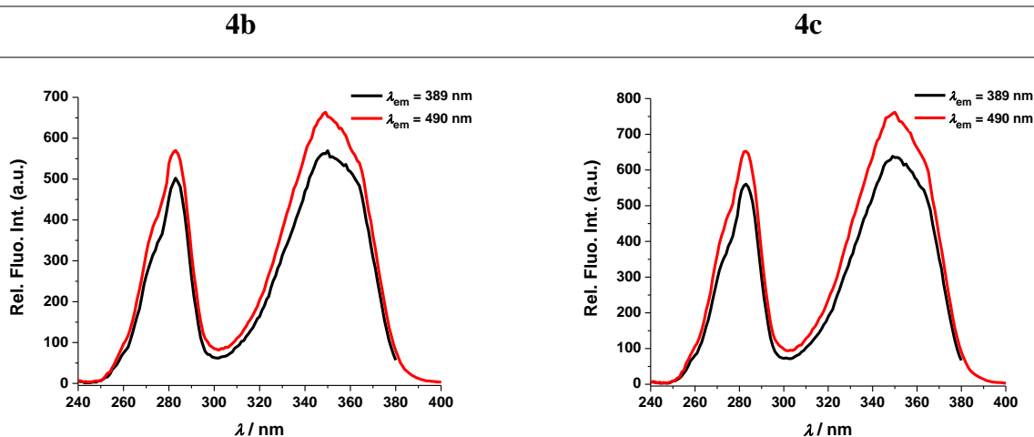
Slika 141. Ekscitacijski spektri spojeva 4b–c ( c = 1,00 \cdot 10^{-6} \text{ mol/dm}^3 in DMSO) snimljeni pri 389 nm (monomerna emisija) i 490 nm (ekscimerna emisija)
