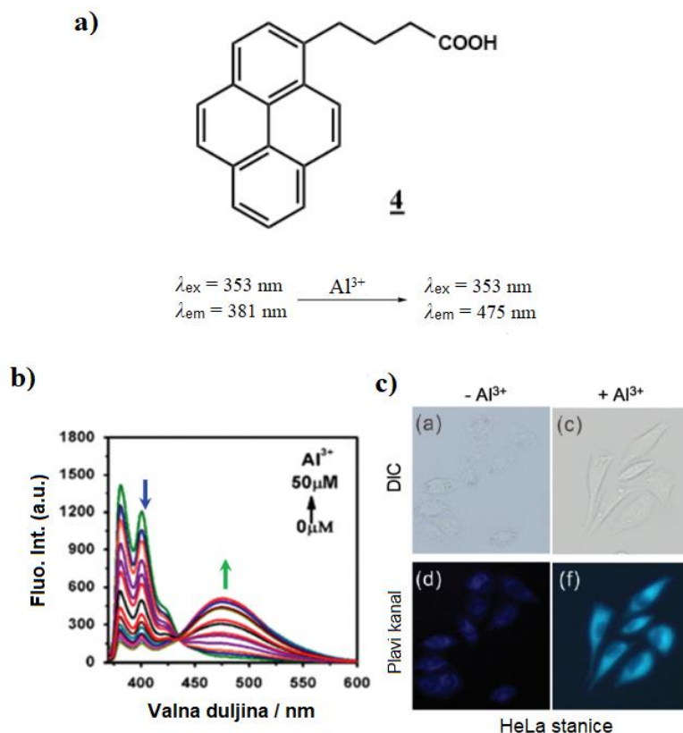
Slika 11. (a) predloženi mehanizam za detekciju iona Al 3+ , (b) promjena fluorescencije spoja 4 u ovisnosti o koncentraciji iona Al 3+ ( \lambda_{\text{ex}} = 353\text{nm} ), (c) primjena spoja 4 za detekciju iona Al 3+ na stanicama HeLa 84
