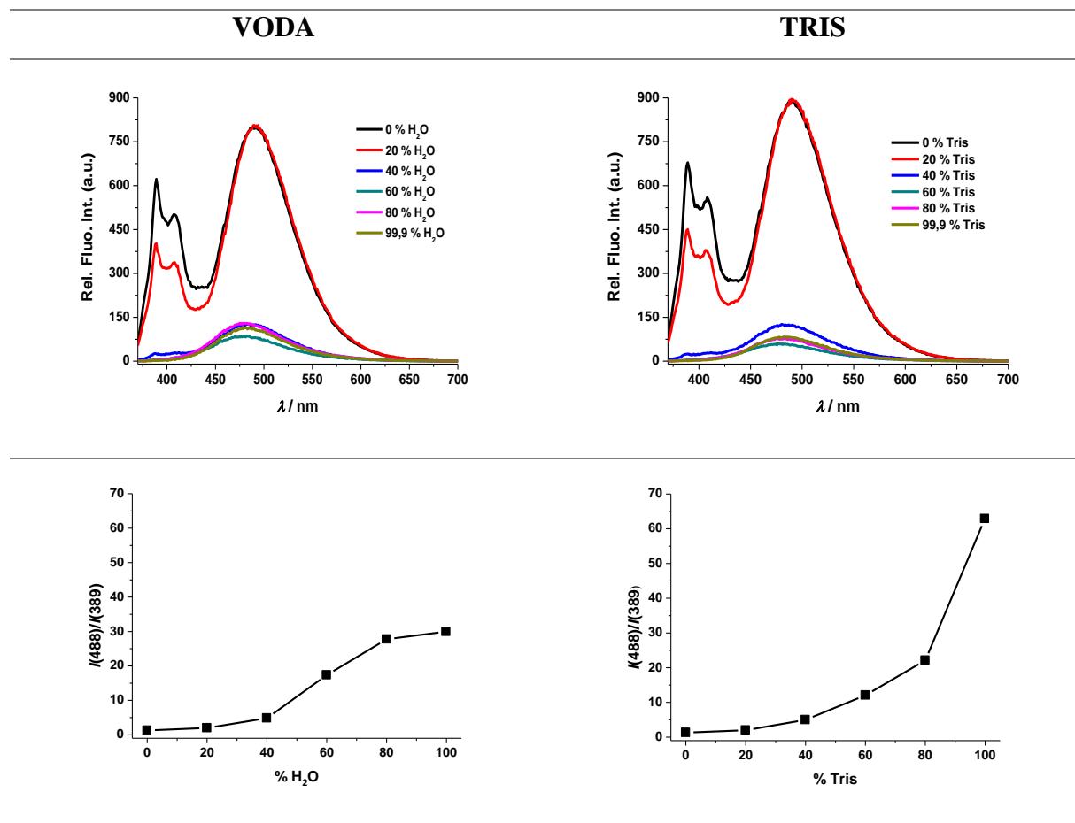
Slika 164. Emisijski spektri ovisnosti fluorescencije spoja 4c ( c = 1,00 \cdot 10^{-6} \text{ mol/dm}^3 ) o udjelu smjese DMSO/H 2 O i DMSO/Tris ( \lambda_{\text{ex}} = 351 \text{ nm} , slit 5 – 5) te odgovarajući omjeri maksimuma fluorescencije ekscimera i monomera
