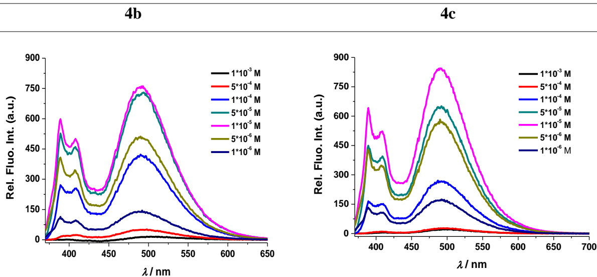
Slika 140. Emisijski spektri koncentracijske odvisnosti fluorescencije spojeva 4b–c ( c = 1,00 \cdot 10^{-6} - 1,00 \cdot 10^{-3} \text{ mol/dm}^3 ) u DMSO ( \lambda_{\text{ex}} = 351 \text{ nm} ; slit 2,5 – 5)
