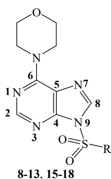
Tablica 6. 1 H NMR pomaci vodikovih atoma 6-morfolinopurinskih derivata.
