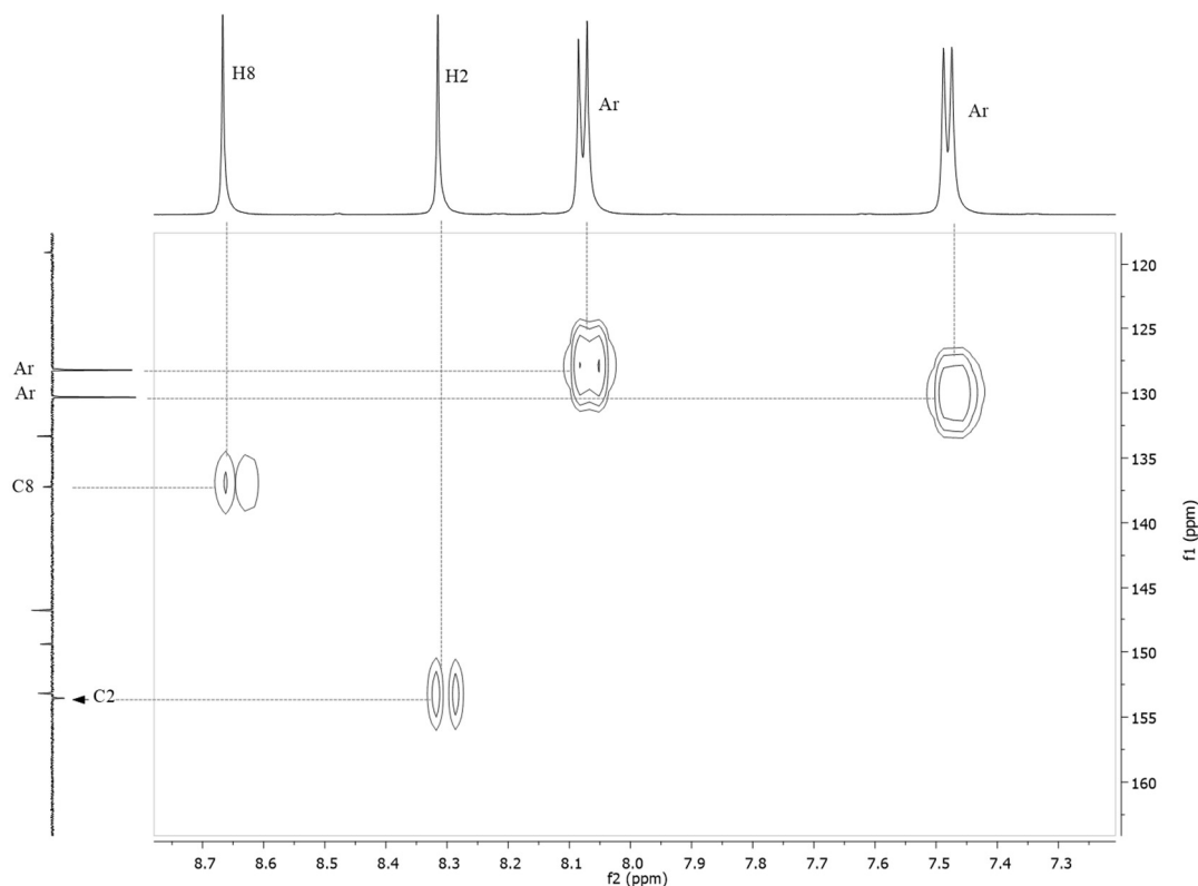
Slika 28. Dio HMQC spektra spoja 8 .
