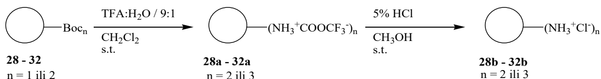
Shema 36. Shematski prikaz pripreme hidrokloridnih soli gvanidinopirolnih derivata 28-32 .
