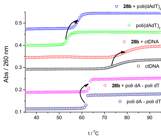
Slika 43. Krivulje mekšanja ct DNA ( \square ), poli dA – poli dT ( \diamond ), poli(dAdT) 2 ( \triangle ) i kompleksa spoja 28b – ct DNA ( \circ ), 28b – poli dA – poli dT ( \triangleleft ) i 28b – poli(dAdT) 2 ( \nabla ) pri omjeru r_{(\text{spoj})/(\text{polinukleotid})} = 0,5 ; \text{pH} = 5 (kakodilatni pufer, I = 0,05\text{ mol dm}^{-3} ).
