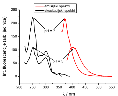
Slika 37. Ekscitacijski (—, \lambda_{\text{em}} = 372 \text{ nm} , \text{pH} = 7,0 i —, \lambda_{\text{em}} = 401 \text{ nm} , \text{pH} = 5,0 ) i emisijski spektri (—, \lambda_{\text{eks}} = 252 \text{ nm} , \text{pH} = 5,0 i \text{pH} = 7,0 ) spoja 28b ( c = 2,0 \times 10^{-6} \text{ mol dm}^{-3} ) u vodi (kakodilatni pufer, I = 0,05 \text{ mol dm}^{-3} ); spektri su korigirani za intenzitet fluorescencije pufera.
