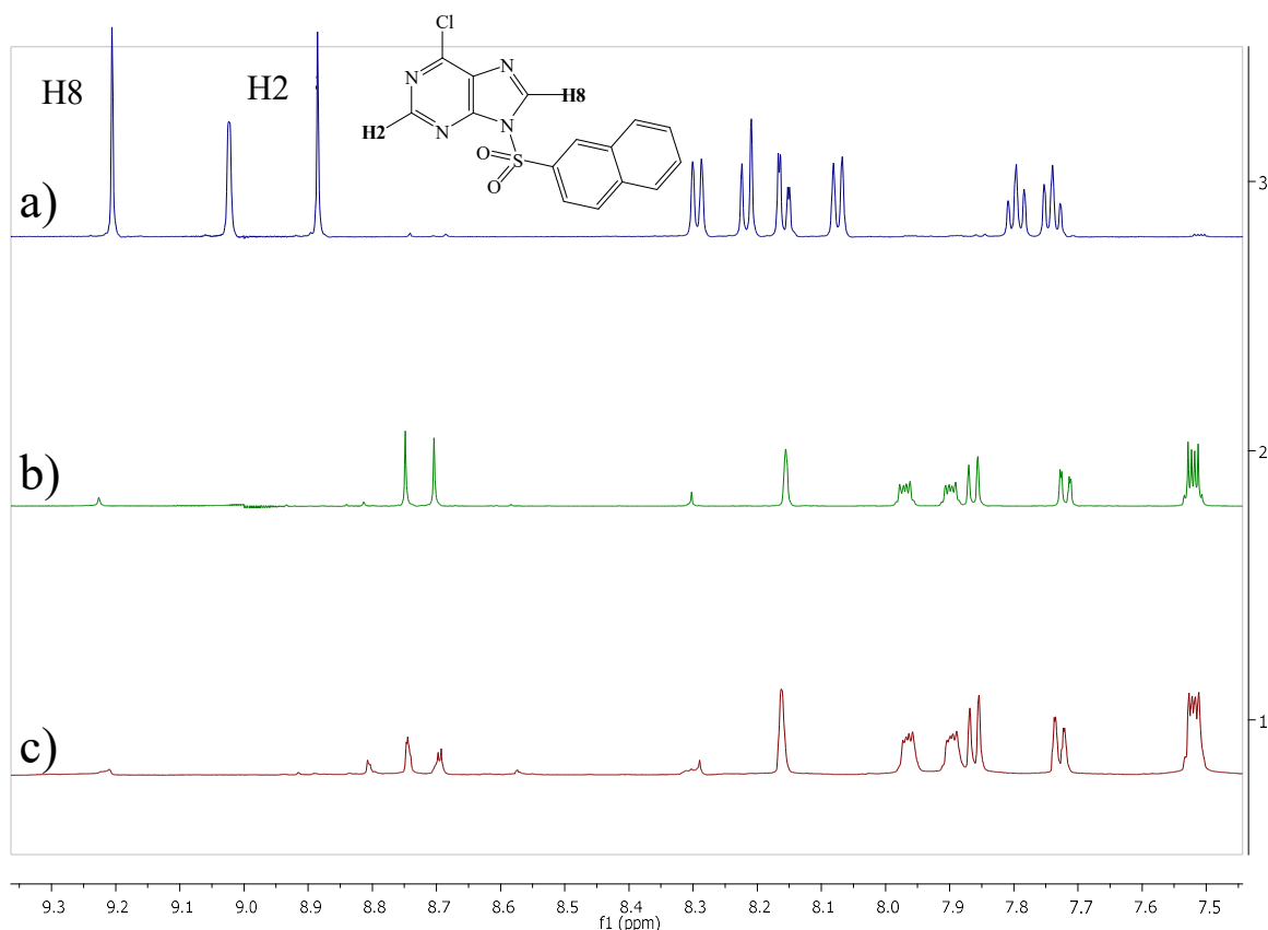
Slika 25. ^1\text{H} NMR spektri spoja 3 u DMSO-u: a) svježa otopina; b) otopina stara 24 sata; c) otopina stara 48 sati.
