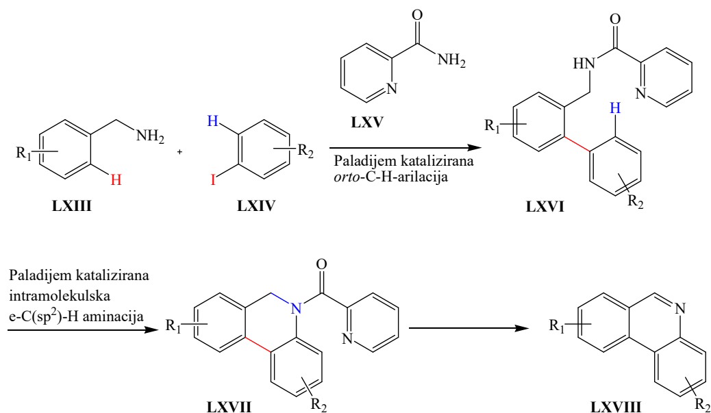
Shema 19. Sinteza fenantridina LXVIII uz paladijev katalizator.
