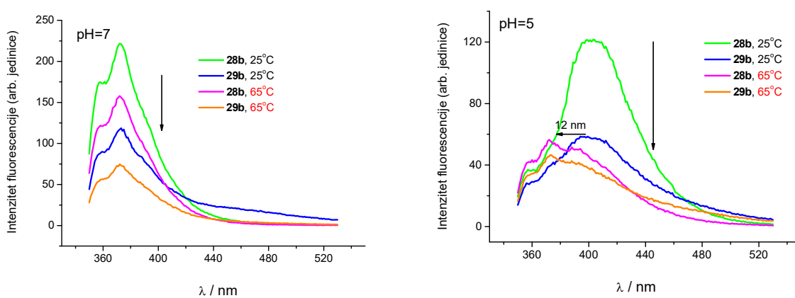
Slika 39. Utjecaj promjene temperature na emisijske spektre spojeva 28b i 29b ( c = 2 \times 10^{-6} mol dm -3 , kakodilatni pufer, I = 0,05 mol dm -3 , pH = 7,0).
