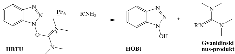
Shema 33. Nastajanje gvanidiliranog nusprodukta.
