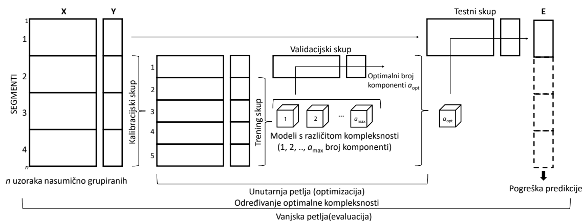
Slika 4.20 Dvostruka unakrsna validacija za optimizaciju i evaluaciju modela. Unutarnjom petljom uzorci u kalibracijskom skupu su nasumično segmentirani u 5 segmenata iz koji se određuje optimalna kompleksnost a_{opt} kao u slici 4.19. Vanjskom petljom uzorci su nasumično segmentirani u 4 segmenta na kojima je razvijen model s a_{opt} brojem komponenti te je izračunata pogreška predikcije modela. Preuzeto i prilagođeno iz [3].
