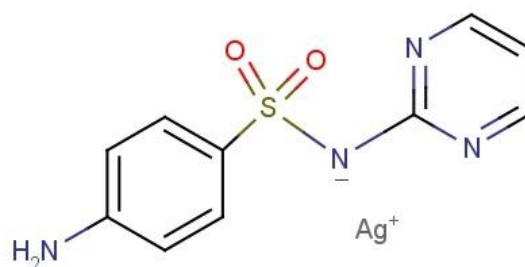
Slika 1. Srebrov(I) sulfadiazin.
