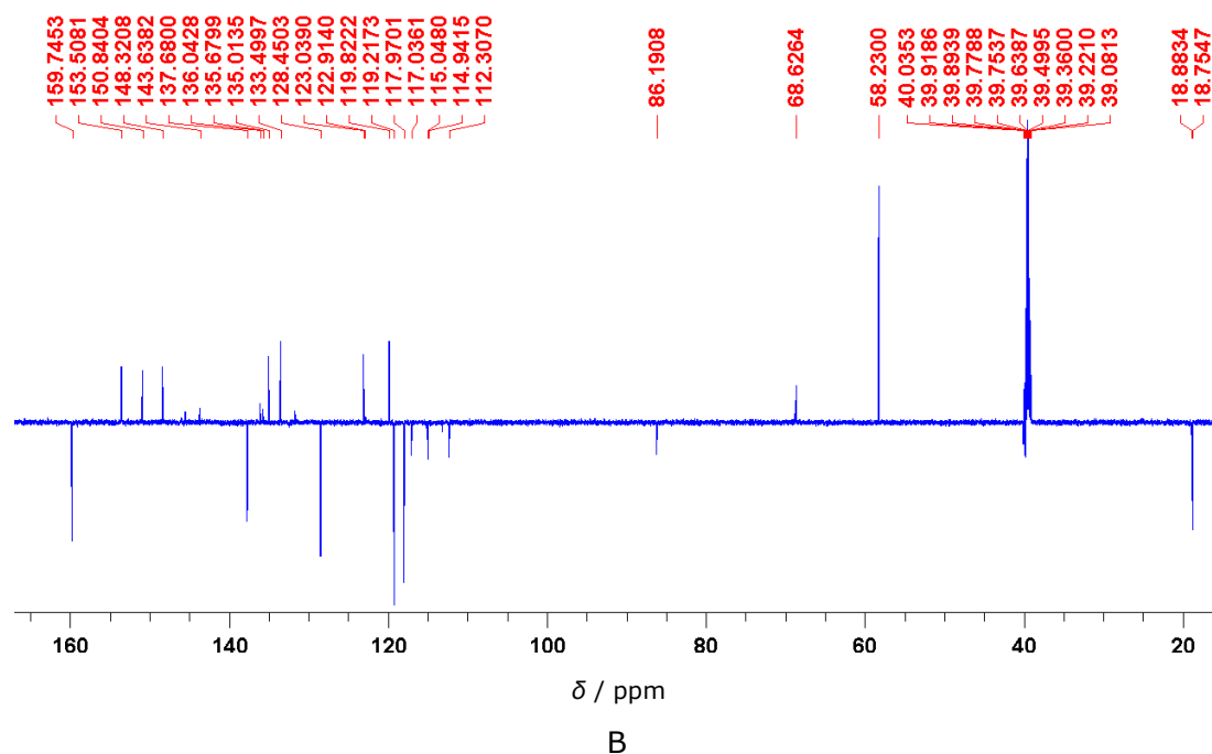
Slika 15. A) 1 H i B) 13 C spektar spoja P3 i P4.
