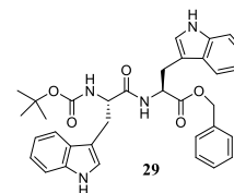
Prilog 43. 1 H NMR (CD 3 OD, 300 MHz) spektar Boc-Trp-Trp-OBn ( 29 )
