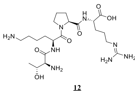
Slika 13. Struktura tuftsina
