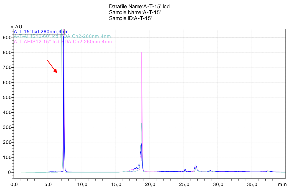
Slika 61. Preklopljeni HPLC kromatogrami dA 10 -dT 10 ozračeno 15 min ( t_R = 7,4 min i 17,5-18,8 min), smjese 36 -dA 10 -dT 10 ozračenih 15 min ( t_R = 7,4 min i 16,5-17 min i 18,8 min) i smjese 36 -dA 10 -dT 10 ozračenih 60 min ( t_R = 7,0 min i 18,6 min i 18,8 min)
