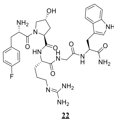
Slika 22. Struktura nemifitida
