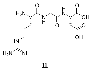
Slika 12. Stuktura RGD-a
