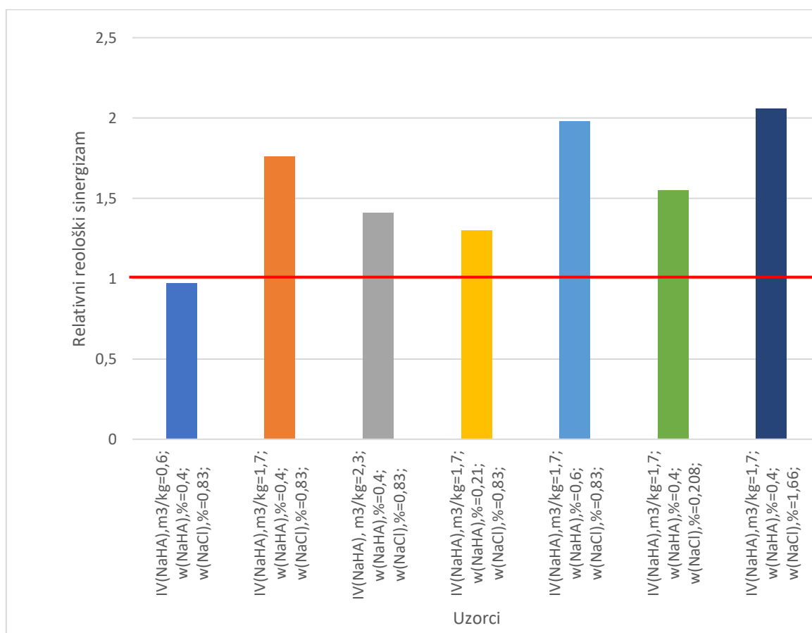
Slika 19.: Relativni reološki sinergizam svih otopina natrijeva hijaluronata različitih intrinzičnih viskoznosti (IV(NaHA), \text{m}^3/\text{kg} ), masenog udjela natrijevog hijaluronatata (w(NaHA), %) i masenog udjela natrijeva klorida (w(NaCl), %)
