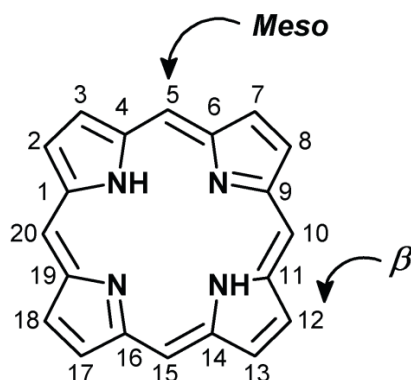
Slika 4. Struktura porfirina (16).
