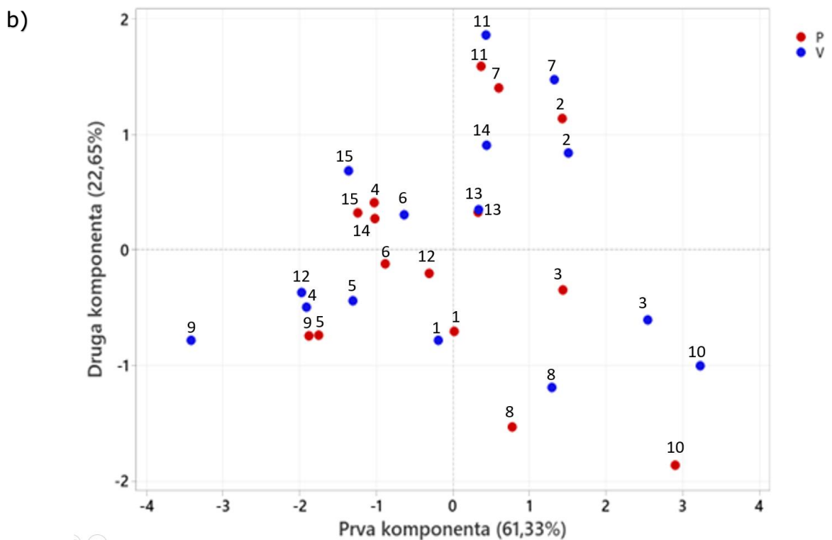
Slika 15 PCA projekcija spektrofotometrijskih testova i svih analiziranih uzoraka vina: projekcija varijabli (a) i uzoraka vina (b) dozrijevanih u podrumu (crveno) i vrulji (plavo) te grupiranje istih u prostoru glavnih komponenti (PC1 i PC2).
