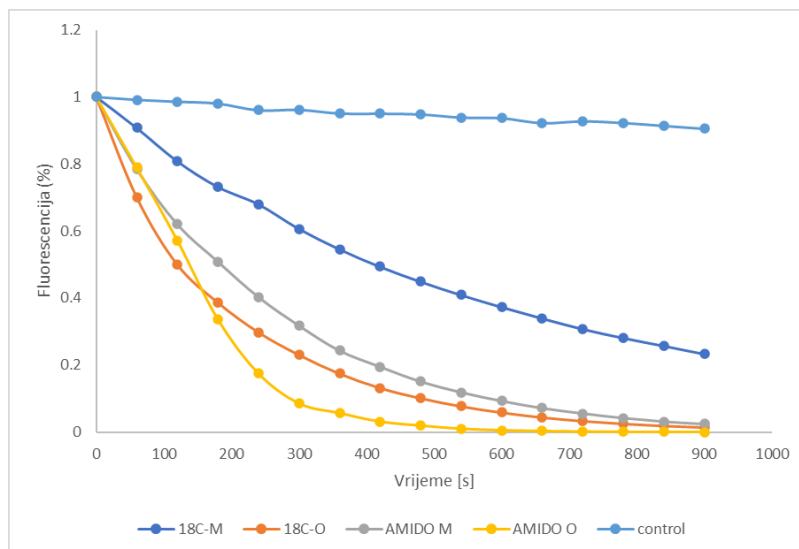
Slika 32: Krivulje dobivene eksperimentom fotodegradacije DPBF-a za određivanje produkcije singletnog kisika ispitivanih N -metiliranih i N -oksidiranih porfirina u etanolu, u odnosu na DPBF kontrolu
