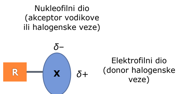
Slika 11. Shematski prikaz anizotropne raspodjele elektronske gustoće oko kovalentno vezanog atoma halogenog elementa u molekuli.
