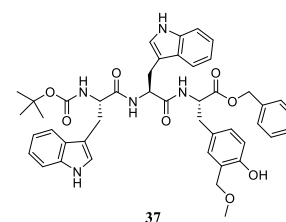
Prilog 58. 1 H NMR (CDCl 3 , 600 MHz) spektar Boc-Trp-Trp-Tyr[CH 2 OCH 3 ]-OBn ( 37 )
