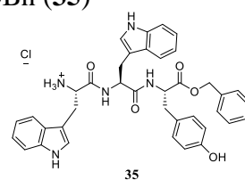
Prilog 54. 1 H NMR (CD 3 OD, 600 MHz) spektar HCl×H-Trp-Trp-Tyr-OBn ( 35 )
