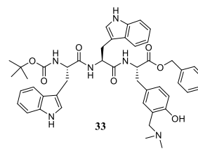
Prilog 50. ^1\text{H} NMR ( \text{CD}_3\text{OD} , 600 MHz) spektr Boc-Trp-Trp-Tyr[ \text{CH}_2\text{N}(\text{CH}_3)_2 ]-OBn (33)
