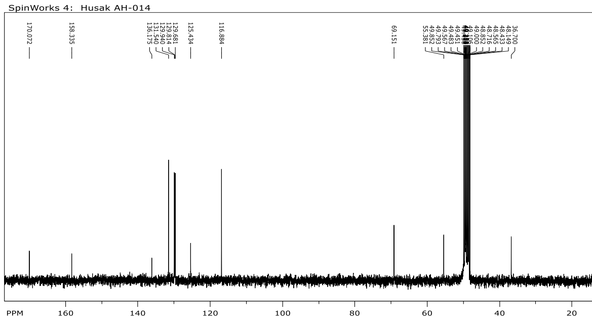
Prilog 18. ^{13}\text{C} NMR ( \text{CD}_3\text{OD} , 75 MHz) spektar \text{TFA}\times\text{H-Tyr-OBn} ( 10 )
