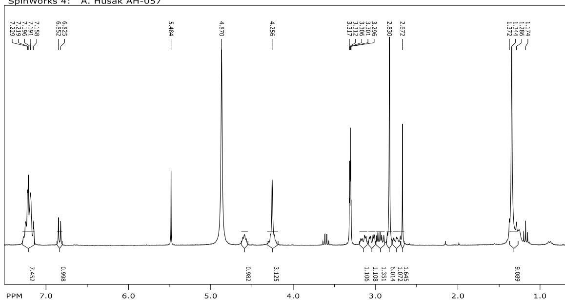
Prilog 26. ^{13}\text{C} NMR ( \text{CD}_3\text{OD} , 150 MHz, APT) spektar Boc-Phe-Tyr[ \text{CH}_2\text{N}(\text{CH}_3)_2 ]-OH ( 18 )
