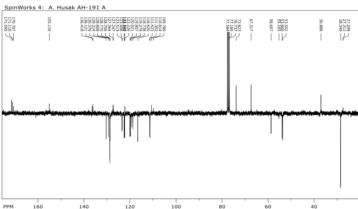
Prilog 59. 13 C NMR (CDCl 3 , 75 MHz) spektar Boc-Trp-Trp-Tyr[CH 2 OCH 3 ]-OBn ( 37 )
