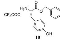
Prilog 17. ^1\text{H} NMR ( \text{CD}_3\text{OD} , 300 MHz) spektar \text{TFA}\times\text{H-Tyr-OBn} ( 10 )
