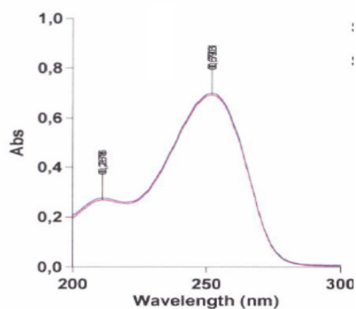
Slika 6. UV spektar metimazola u 0,1 N H 2 SO 4 .
