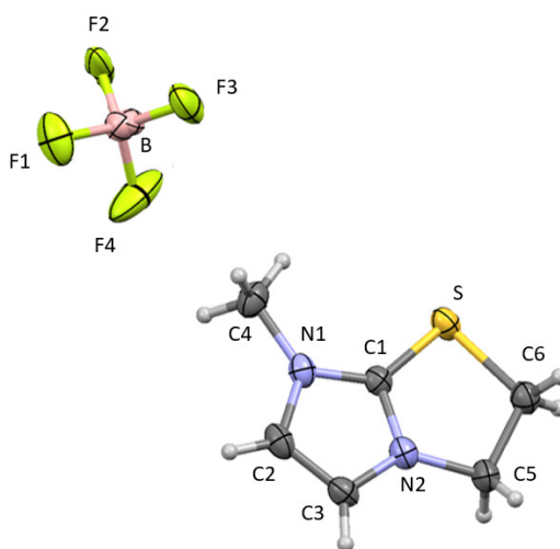
Slika 69. Molekularna struktura 7b sa shemom atomskog numeriranja.
