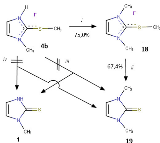
Shema 22. Pokus direktne metilacije i demetilacije 4b , i ) \text{CH}_3\text{I} , \text{MeCN} , \text{NaHCO}_3 , refluks, 5h; ii ) \text{NaHCO}_3 , \text{MeCN} , refluks 13h; iii ) \text{NaHCO}_3 , \text{MeCN} , refluks, 8h; iv ) \Delta (147°C, 2h).
