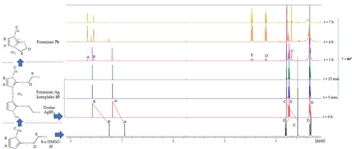
Slika 28. 1 H NMR spektri transformacije 6 u 10 i 7b .
