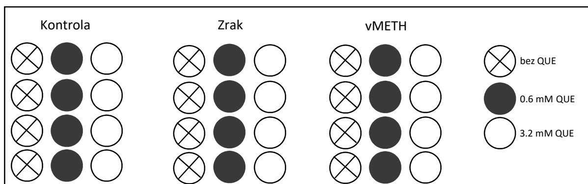
Slika 4. Dizajn eksperimenta. Eksperiment se sastojao od tri skupine; KONTROLA =netretirani mušjaci (n=12), ZRAK = mušjaci koji su primili vrući zrak u FlyBong -u (n=12) i vMETH = mušjaci koji su primili 1 dozu vMETH na 1 min (n=12). U svakoj skupini su bile tri podskupine različitih koncentracija QUE pomiješanog u hranu: križić= hrana bez QUE, crni krug= 0.6 mM QUE i bijeli krug= 3.2 mM QUE. Svakom mušjaku je dodana djevnica koja nije bila prethodno tretirana. Mušice su ostavljene na hrani 6 dana. n=broj mušjaka.
