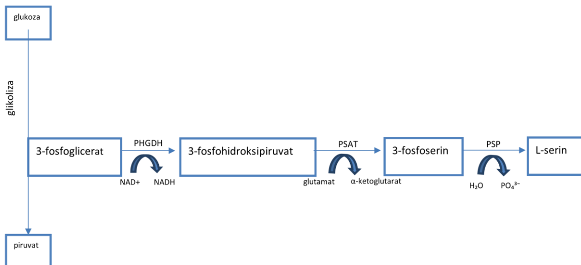
Slika 3: Shematski prikaz puta biosinteze serina.
