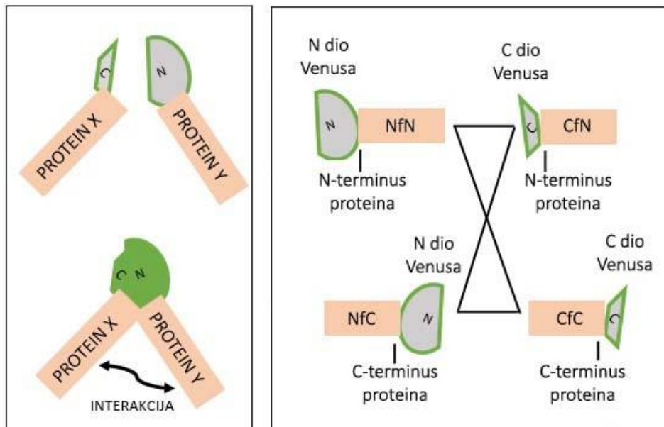
Slika 12. Lijevo: Pojednostavljena shema komplementacije N- i -C dijela proteina Venusa nakon interakcije proteina X i Y s kojima su fuzionirani. Desno: Shematski prikaz načina označavanja Venusa konstrukata u sve 4 topologije. Prvo slovo označava dio Venusa, slovo „f“ označava riječ fuzioniran, treće slovo označava na kojem kraju proteina se nalazi Venusa: NfN = N dio Venusa fuzioniran na N-terminus
