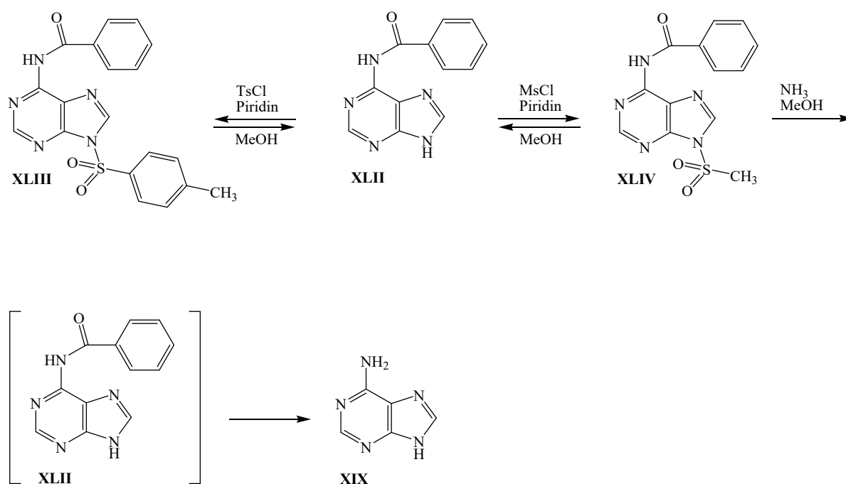
Shema 12. Ispitivanje stabilnosti sulfoniliranih spojeva na primjeru N 6 -benzoidadenina XLII.
