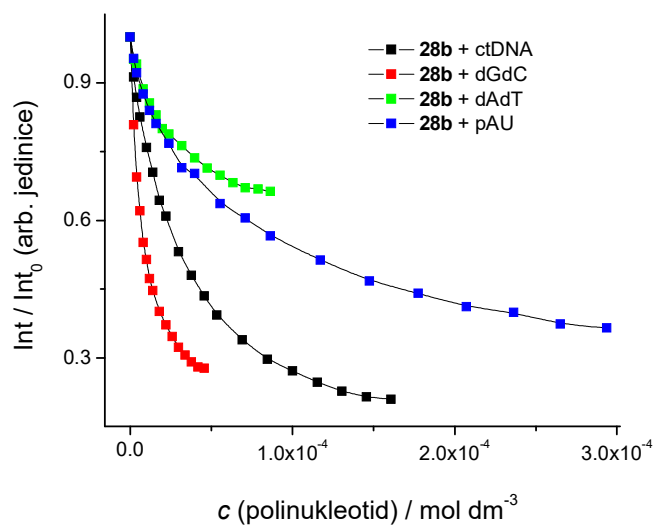
Slika 42. Promjene intenziteta emisije spoja 28b ( c = 2 \times 10^{-6} mol \text{dm}^{-3} ; \lambda_{\text{eks}} = 300 nm, pH = 5,0) prilikom titracija s ctDNA (—■—), poli A – poli U (—■—), poli(dAdT) 2 (—■—) i poli(dGdC) 2 (—■—).
