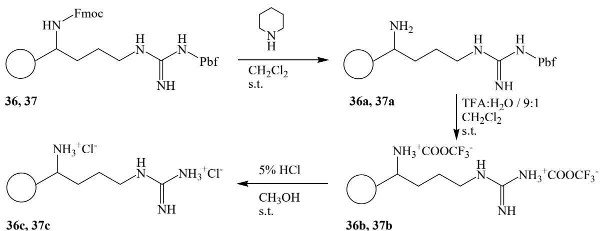
Shema 37. Shematski prikaz priprave hidrokloridnih soli argininskih derivata 36c i 37c .
