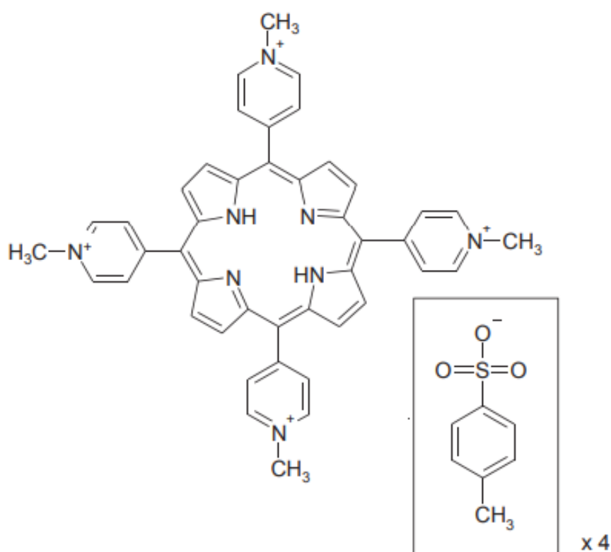
Slika 6: Kemijska struktura TMPyP-a. (41)
