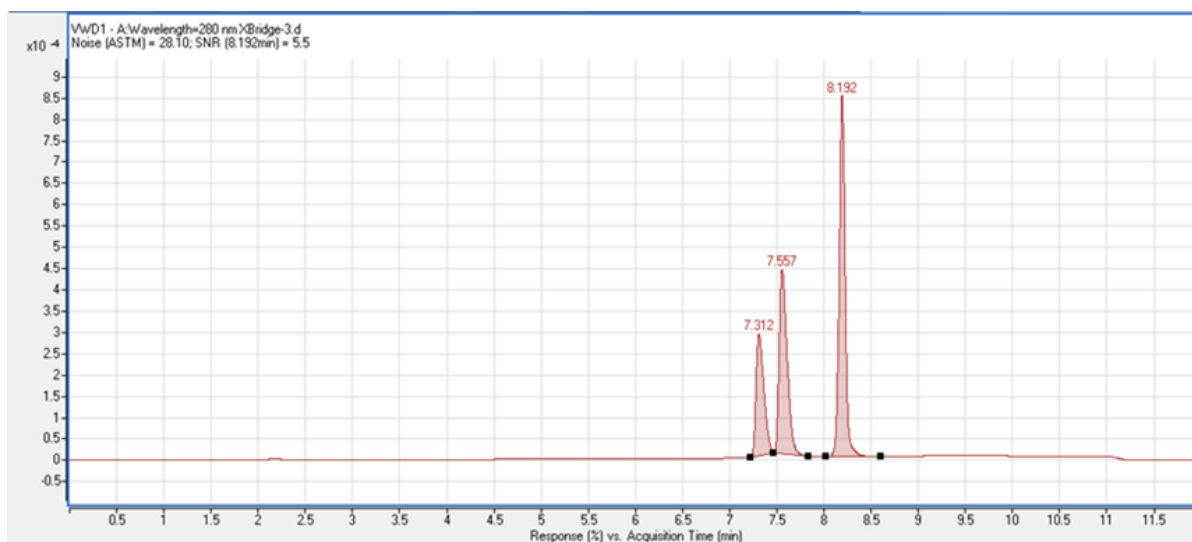
Slika 11 Kromatogram identifikacijske otopine dobiven na koloni XBridge C18 3,5 \mu\text{m} , 150 x 4,6mm
